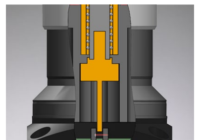
A guia linear montada em rolamento de esferas permite baixas forças de medição
