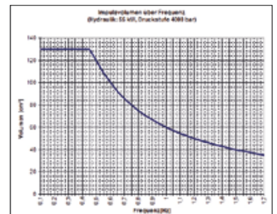
频率与当量关系图
